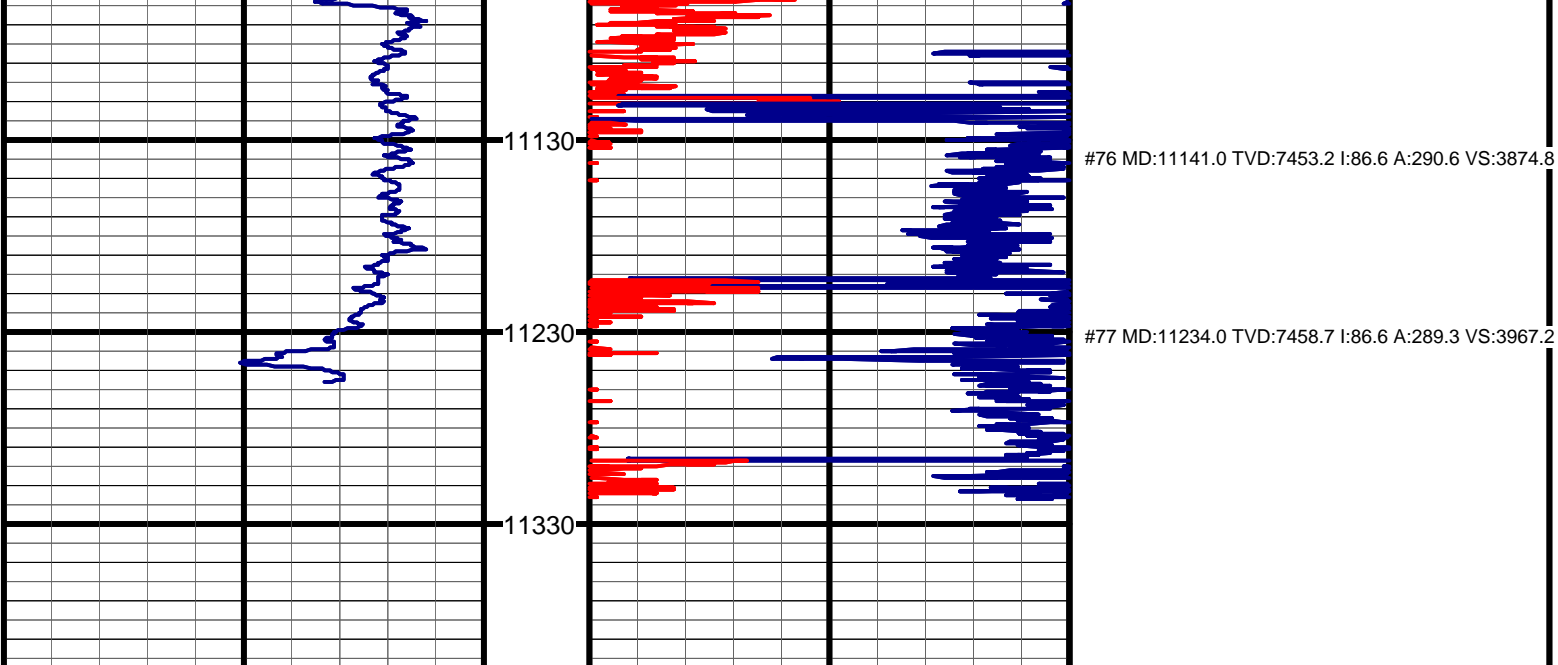
Gamma API (MD) Track: 1 API
