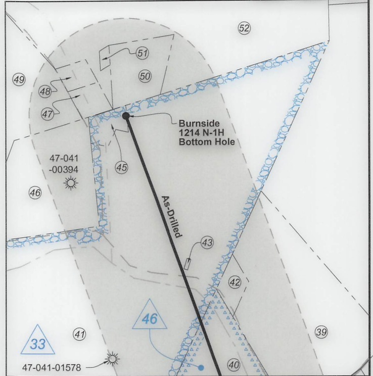
Detail 3 - Scale: 1" = 500"
